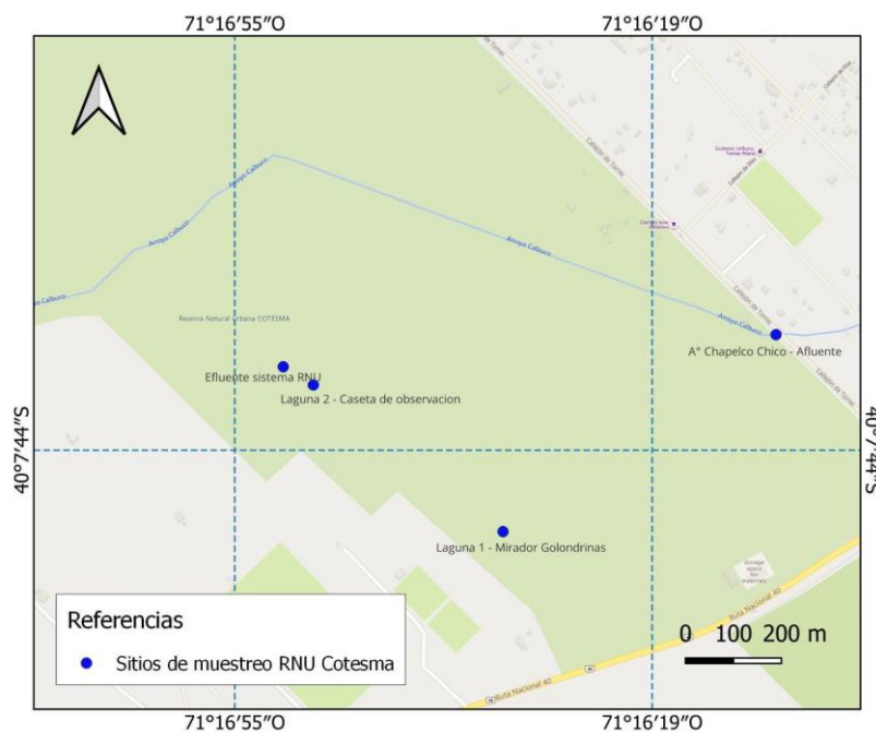
Fig 1: Mapa del área de la RNU Cotesma y su sistema hídrico: Afluente A° Chapelco Chico (sitio 1), laguna 1 Mirador Golondrinas (sitio 2), laguna 2 Caseta de observacion (sitio 3) y efluente del sistema RNU (sitio 4)
